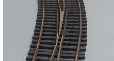
K-Gleis Peco Code 100 IBW r 2251 / 64,6mm 2251 bewegl. Herzstück
