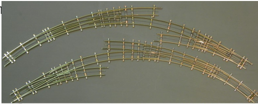
Gleisverbindungen K-Gleis von R3 nach Zwischenradius 3/4 Ausführung Schattenbahnhof
