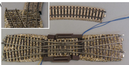
Märklin Metallgleis DKW Geometrie Modellgleis Peco-Spulenansätze und Polarisierung mit Relais
