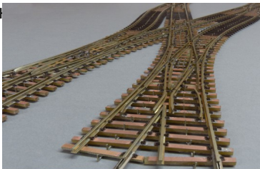
K-Gleis doppelte Gleisverbindung individuelle Gleisabstände Kleineisen aus Weinert mein Gleis
