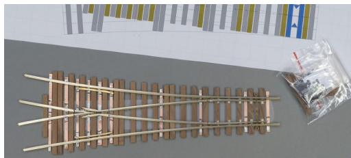
Spur 0 Code 143 ABW Halbbausatz Geometrie 2 x 45025
