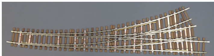
Spur 0 Lenz Code 143 Doppelinnenbogenweiche individuell, Basis Lenz 45044
